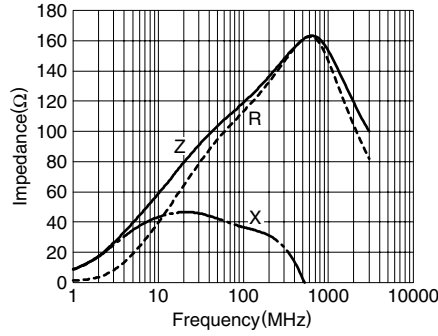
MMZ1005S121C
