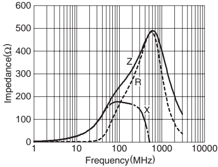
MMZ0603Y241C
