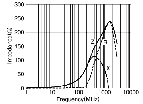
MMZ1005D241C
