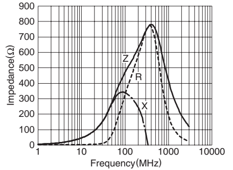
MMZ0603Y471C
