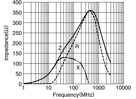
MMZ1005S241C
