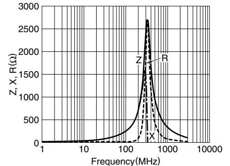
MMZ1005D241C
